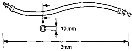
Empfohlener Einführungsschlauch
