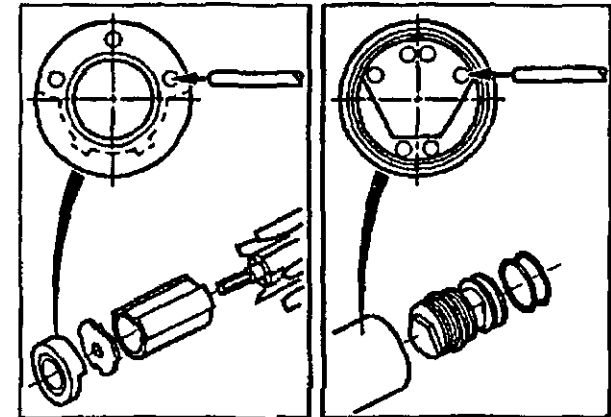
Pour le Montage: Moteur assemblé, se référer à l'illustration principale
