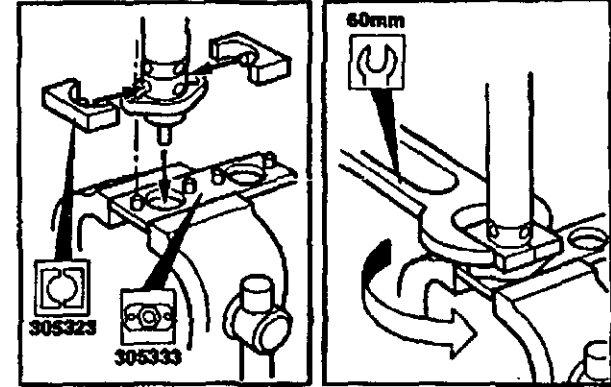
Pour le Démontage: Se référer à l'illustration principale
