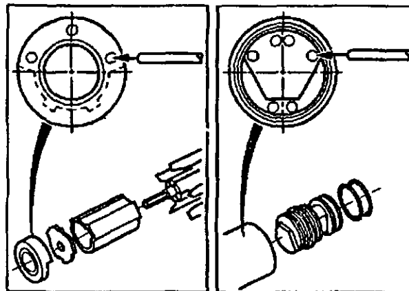
Pour le Montage: Moteur assemblé, se référer à l'illustration principale
