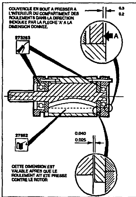
Pour le Montage: Moteur assemblé, se référer à l'illustration principale
