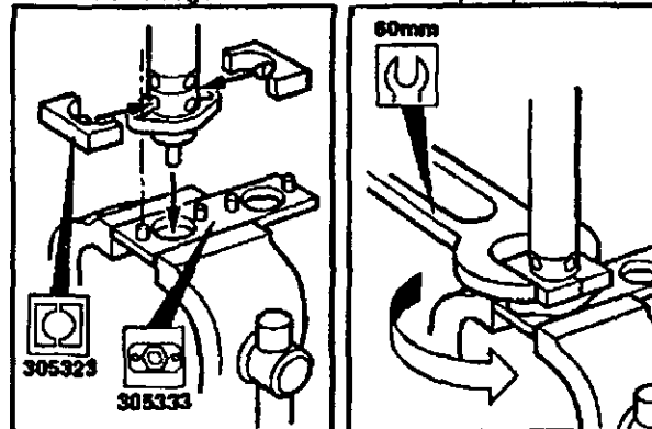
Pour le Démontage: Se référer à l'illustration principale
